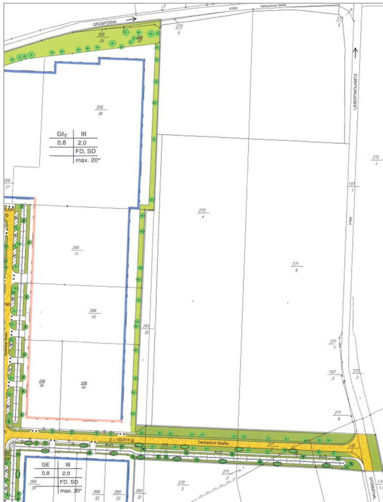
Abb. 3 Auszug Planteil B-Plan „Gewerbegebiet Störmthal Nord 1.1 - 3. Änderung“
